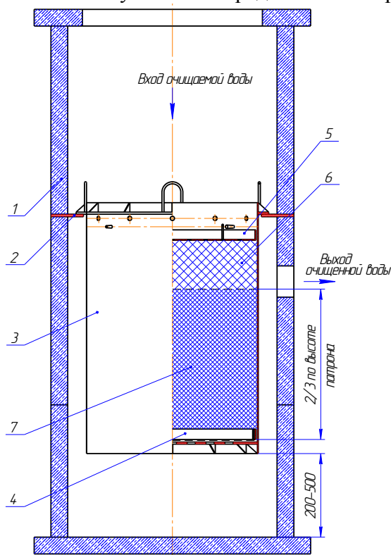
Рис. 1. 1 – Бетонный колодез. 2 – Опорное кольцо. 3 – Комбинированный патрон. 4 – Нижняя решетка. 5 - Верхняя решетка. 6 – Механическая загрузка патрона (синтепон с лавсаном – 1/3 по высоте патрона). 7 – Угольный сорбент (2/3 по высоте патрона).
