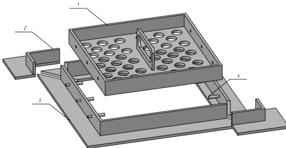
Рис. 1. Люк обслуживания специальный – комплект (крепеж не показан)
